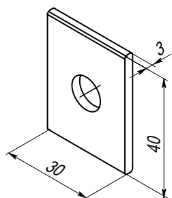
Шайба 30x40 (алюм.) Отверстие Ø 11мм
