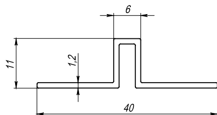
Профиль вертикального шва (алюм.)
