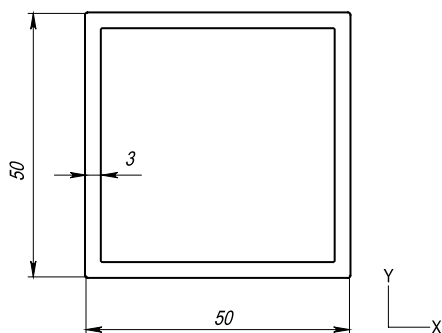
Профиль вспомогательный (алюм.)
